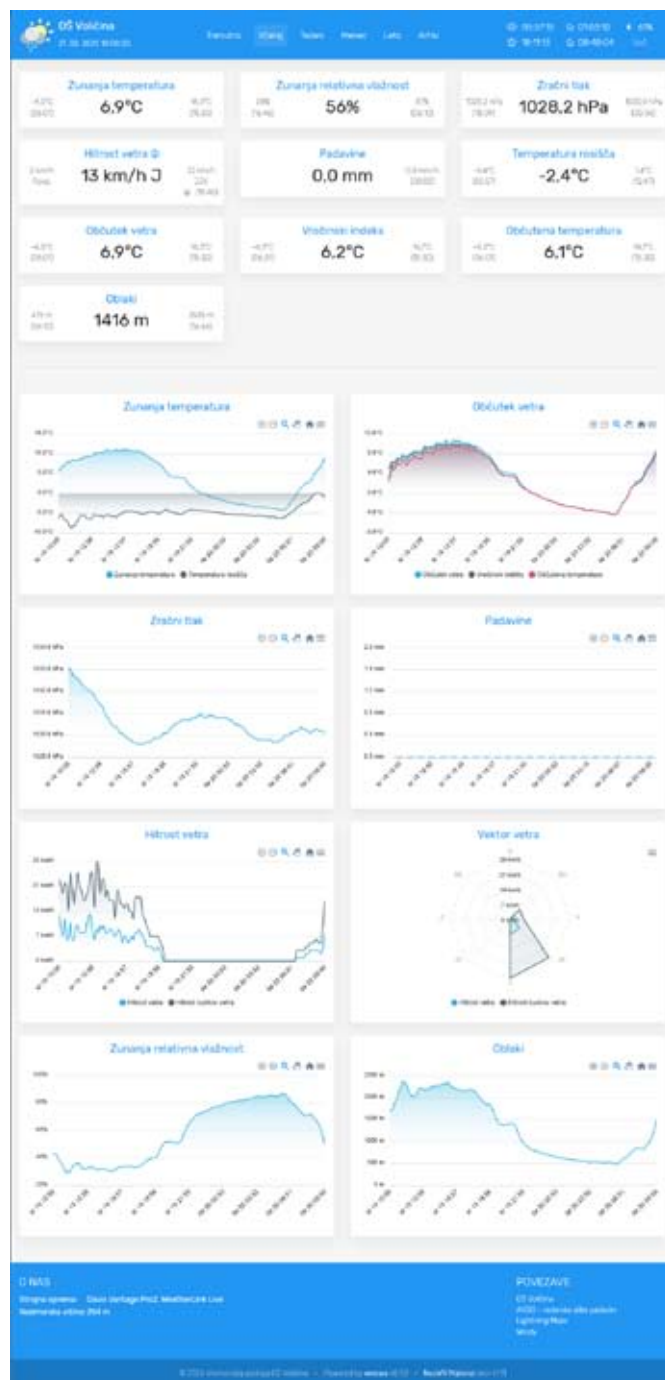
Primer pregleda vremenskih podatkov v okolju WeeWX za merilno postajo OŠ Voličina za 21. 3. 2025
