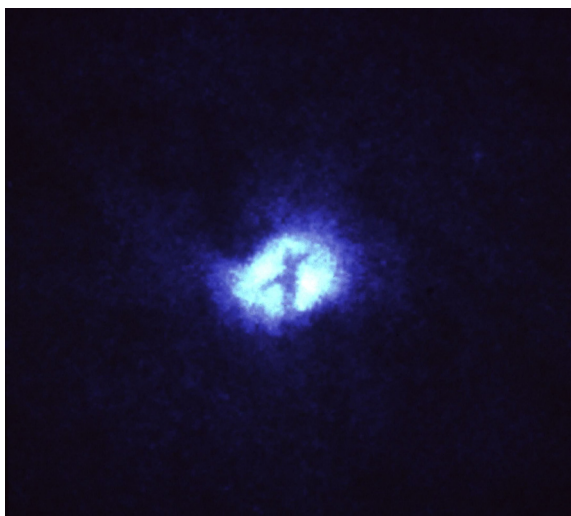
Jedro galaksije Vrtinec, kjer križ dveh prašnih obročev kaže na prisotnost črne luknje.
